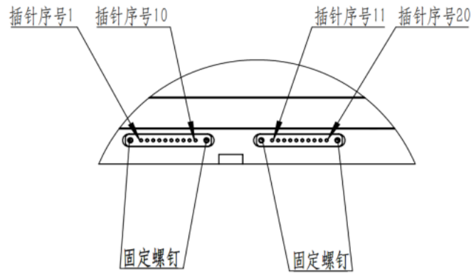
线序定义
